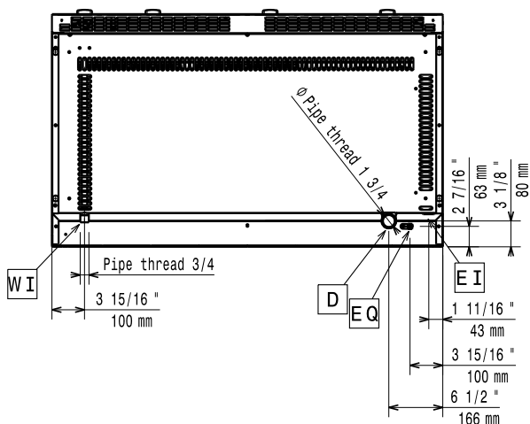
Planta
